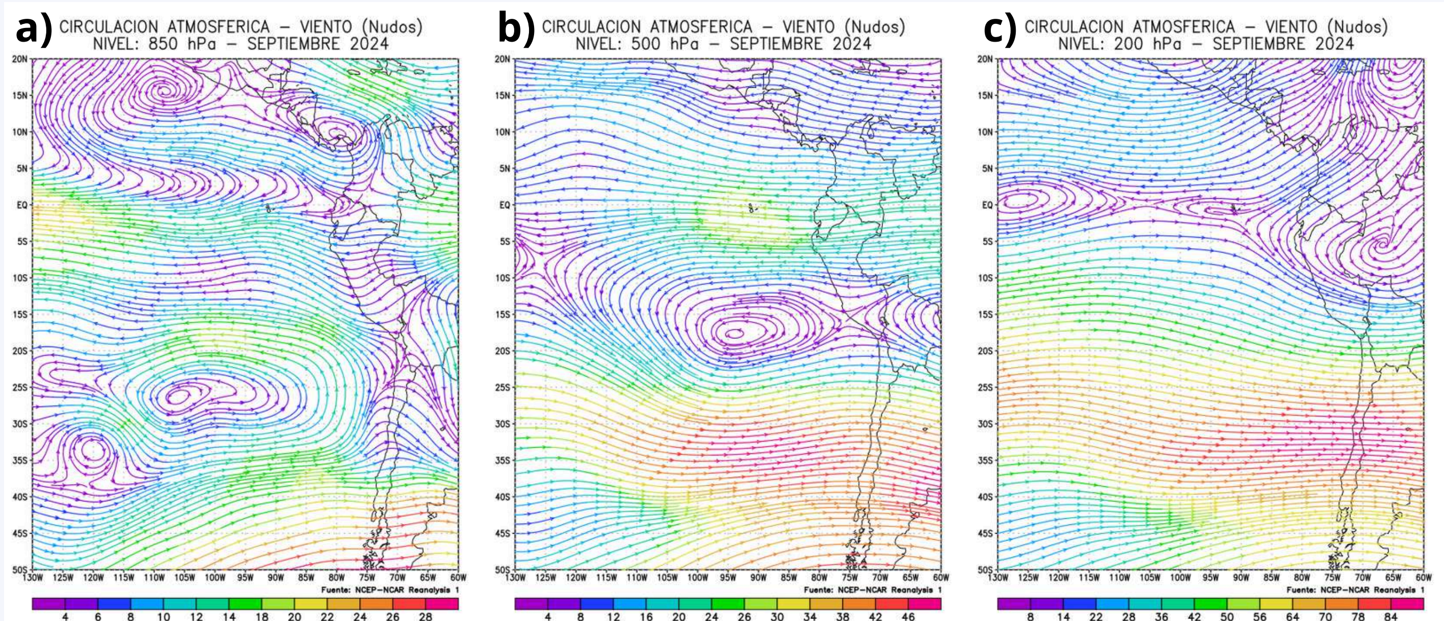
Figura 7. Promedio mensual de la circulación atmosférica del viento (nudos) a) 850hPa, b) 500hPa y c) 200hPa en la región ecuatorial oriental entre los 20°N-50°S y 140°W-060°W. Periodo: setiembre 2024. Fuente: NCEP/NCAR. Elaboración: DIHIDRONAV.
