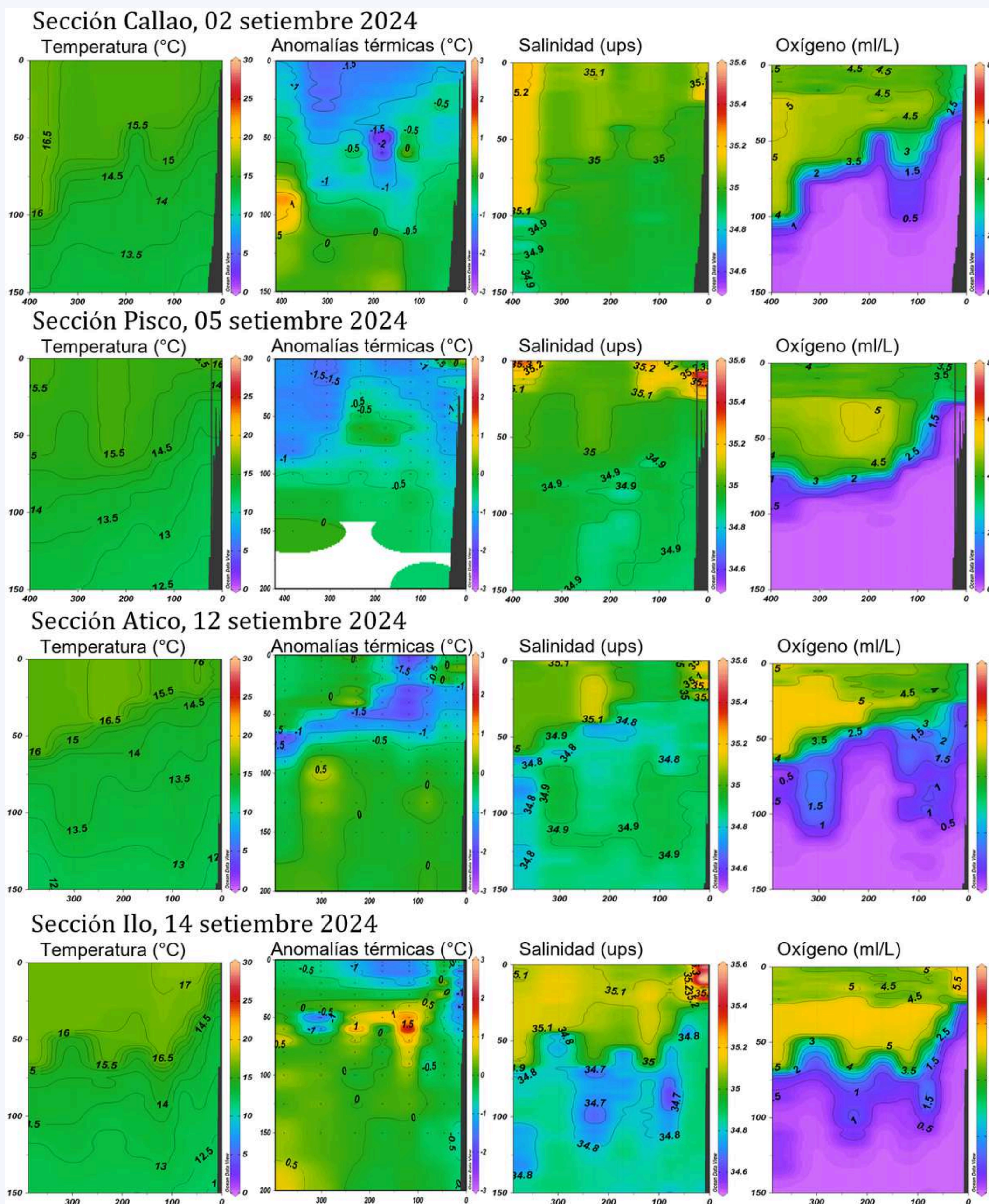
Figura 13. a) Perfiles de temperatura, anomalía de temperatura, salinidad y oxígeno disuelto frente a Callao (02 setiembre), Pisco (05 setiembre), Atico (12 setiembre) e Ilo (14 setiembre), provenientes del crucero oceanográfico 1024 realizado por La Marina de Guerra del Perú entre el 02 y 14 de setiembre de 2024. Fuente y procesamiento: DIHIDRONAV.
