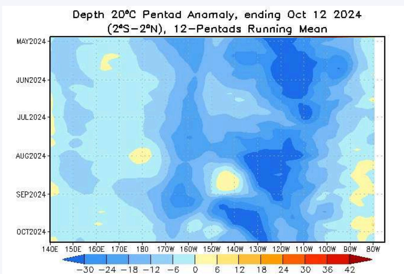
Figura 6. Diagrama longitud-tiempo de la anomalía de la profundidad de la isoterma de 20^{\circ}\text{C} (m) entre los 02^{\circ}\text{N}-02^{\circ}\text{S} . Periodo: mayo- octubre 2024. Fuente: NOAA.
