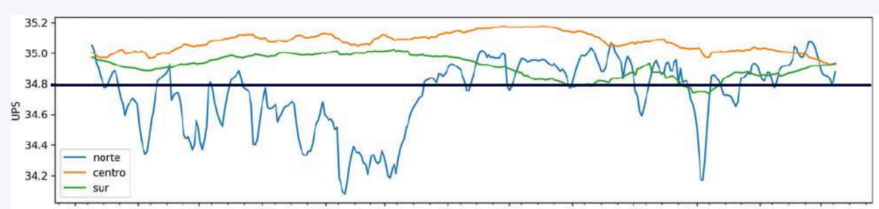
Figura 14. Promedio diario de a) temperatura superficial del mar (°C), b) anomalía de la TSM (°C), c) anomalía de nivel medio del mar (cm), y d) salinidad del mar (PSU) (la línea negra indica el vaor de 34.8PSU; frente a la costa de Perú. Periodo: octubre 2023 - octubre 2024.
