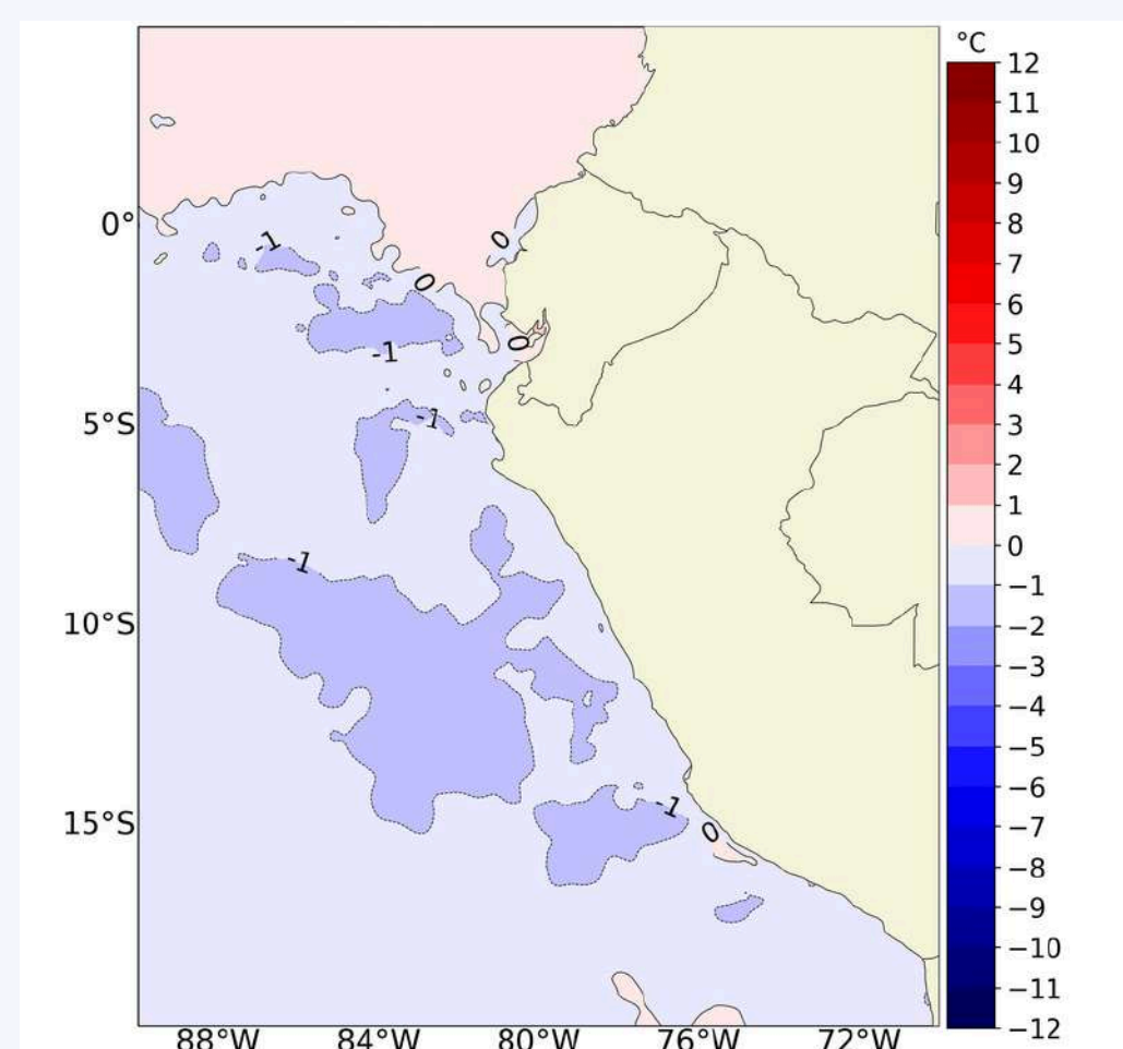
Figura 8. Anomalía de la Temperatura superficial del mar en la región oriental. Periodo: setiembre 2024. Fuente: OSTIA. Elaboración: DIHIDRONAV.
