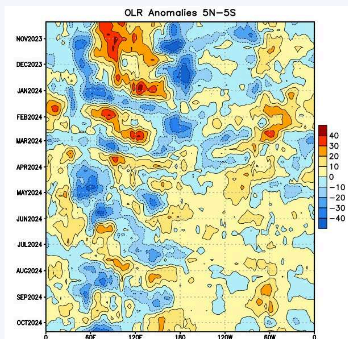
Figura 1. Promedio de la anomalía de radiación de onda larga en la región ecuatorial entre los 05°N-05°S. Periodo: octubre 2023 al 12 de octubre 2024. Fuente: NOAA.
