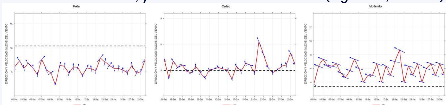
Figura 16. Series de la velocidad del viento y su dirección predominante frente a Paíta, Callao y Mollendo (izquierda a derecha). Período: setiembre 2024. Fuente y elaboración: DIHIDRONAV.
