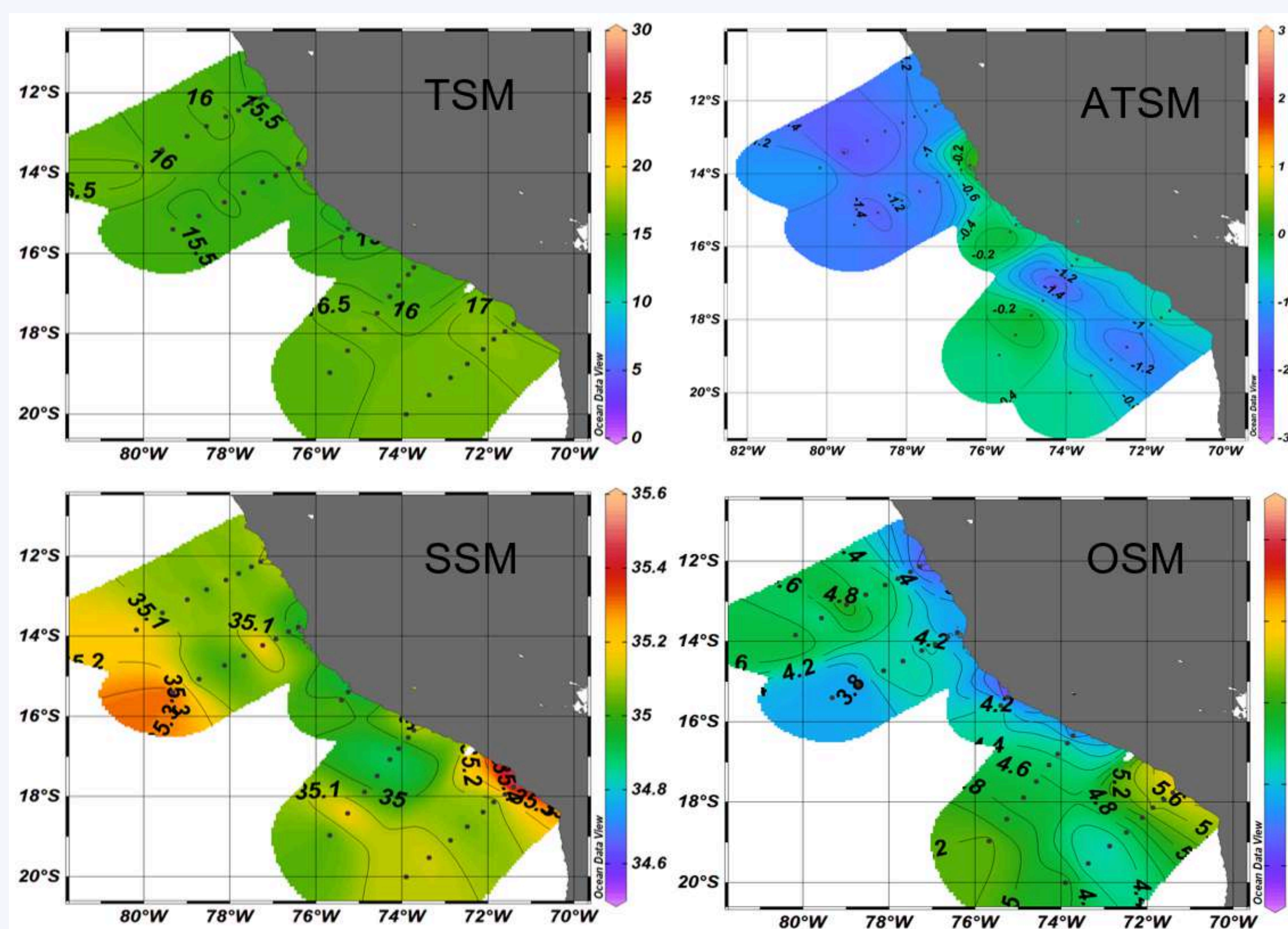
Figura 12. Temperatura superficial del mar, anomalía de la TSM*, Salinidad superficial del mar, y oxígeno disuelto en la superficie frente a la costa sur de Perú, provenientes del crucero oceanográfico 1024 realizado por La Marina de Guerra del Perú entre el 02 y 14 de setiembre de 2024. Fuente y procesamiento: DIHIDRONAV.
