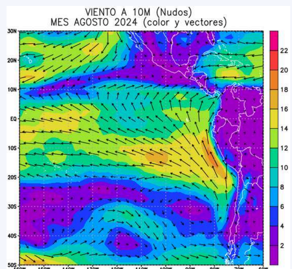
Figura 10. Promedio mensual de la velocidad del viento a nivel del mar en la región oriental. Periodo: agosto 2024.
