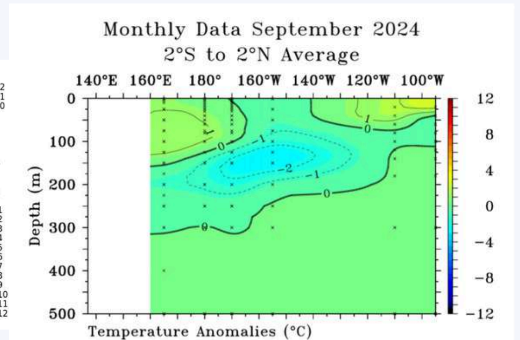
Figura 5. Promedio mensual de la anomalía de la temperatura subsuperficial del mar en la región ecuatorial entre los 02°N-02°S. Periodo: setiembre 2024. Fuente: NOAA.
