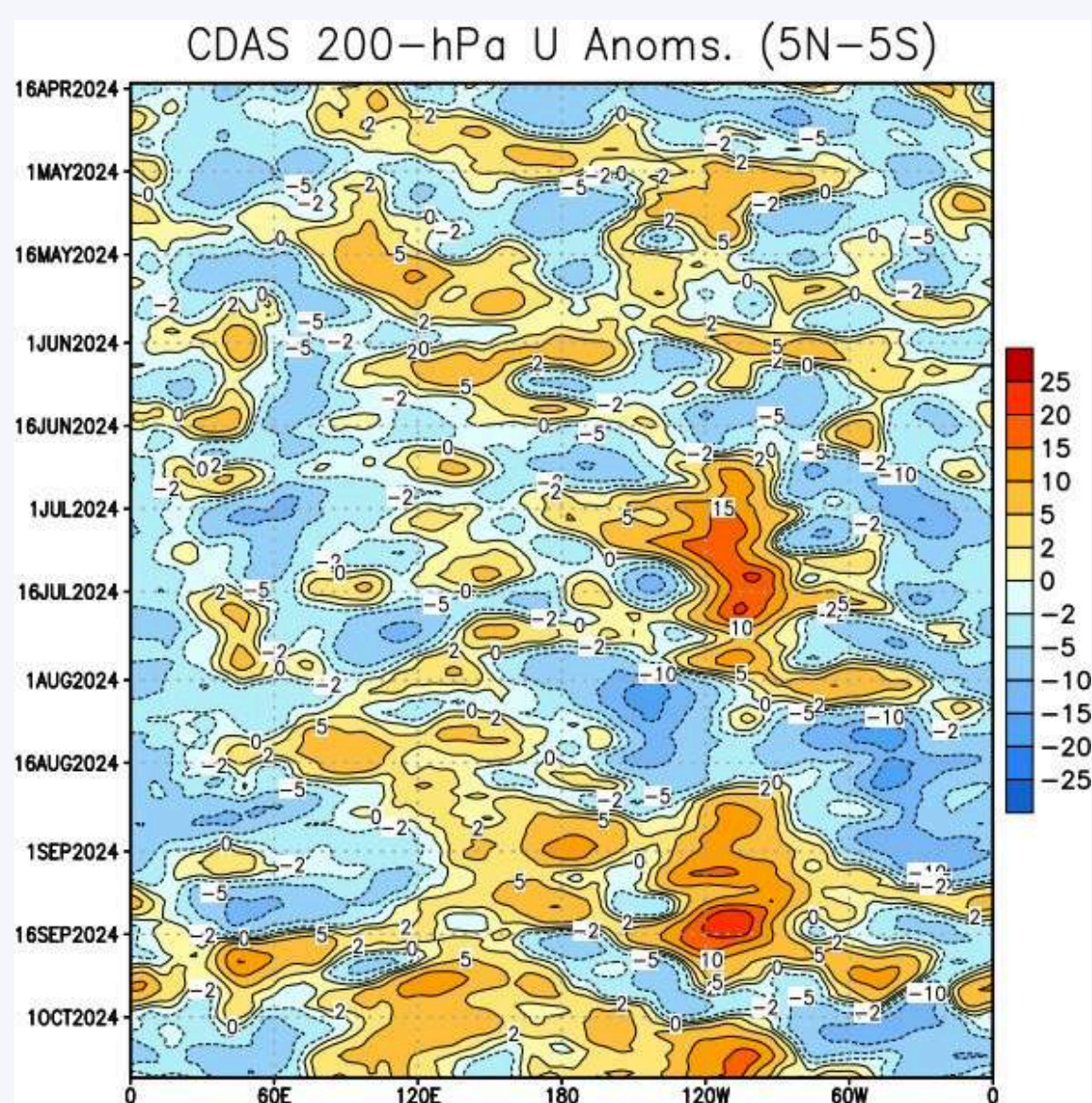
Figura 2. Promedio de la anomalía de vientos zonales a 850hPa en la región ecuatorial entre los 05°N-05°S. Periodo: abril 2024 al 12 de octubre 2024. Fuente: NOAA.
