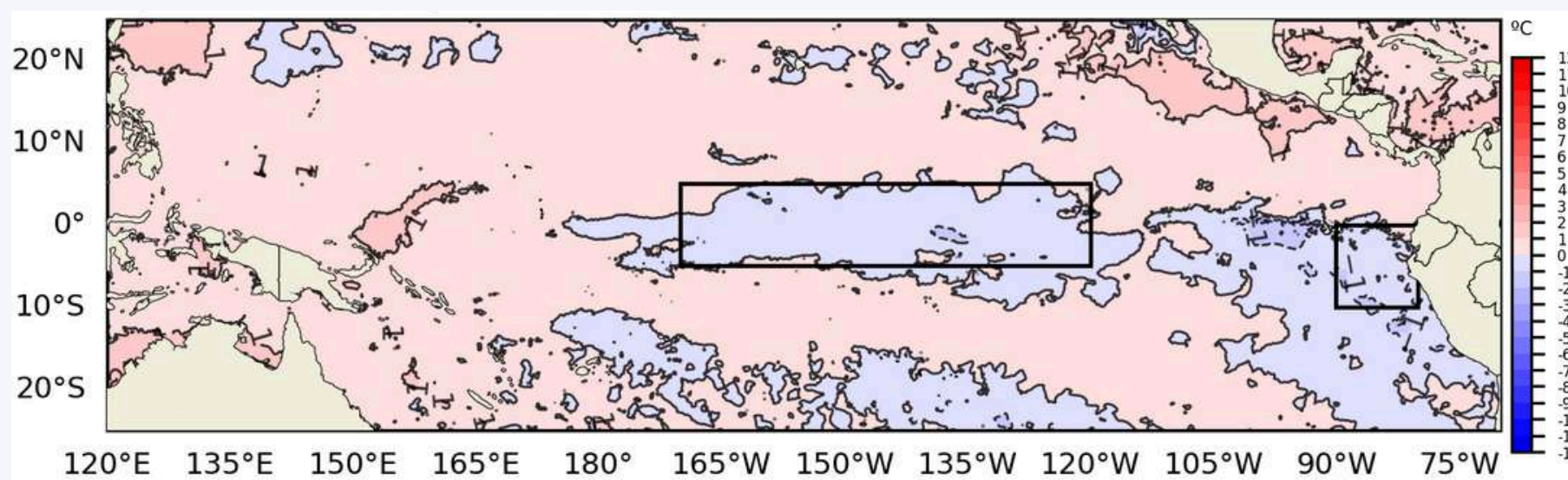
Figura 4. Promedio mensual de la anomalía de la temperatura superficial del mar en la región ecuatorial entre los 25°N-25°S. Periodo: setiembre 2024. Fuente: OSTIA. Elaboración: DIHIDRONAV.
