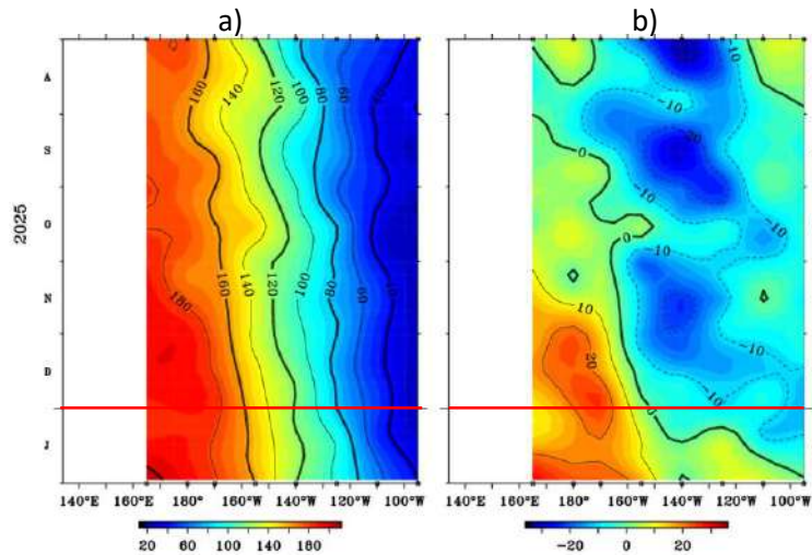
Figura 1.3.2. Diagrama longitud-tiempo de la a) profundidad de la isoterma de 20°C (m) y b) anomalía de la profundidad de la isoterma de 20°C (m) (02°N – 02°S). Periodo: agosto 2025 – enero 2026. Fuente: TAO/TRITON, PMEL/NOAA.
