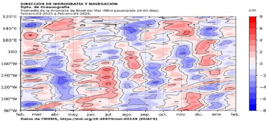
Figura 1.4.1. Diagrama de Hovmöller de la anomalía del nivel del mar en la región ecuatorial (cm), entre los 120°E-080°W (02°N - 02°S) con filtro pasa banda de 10-60 días. Periodo: 01 de febrero 2025 – 01 de febrero 2026. Fuente: GODAS, Climatología 1991–2020. Procesamiento: DIHIDRONAV.
