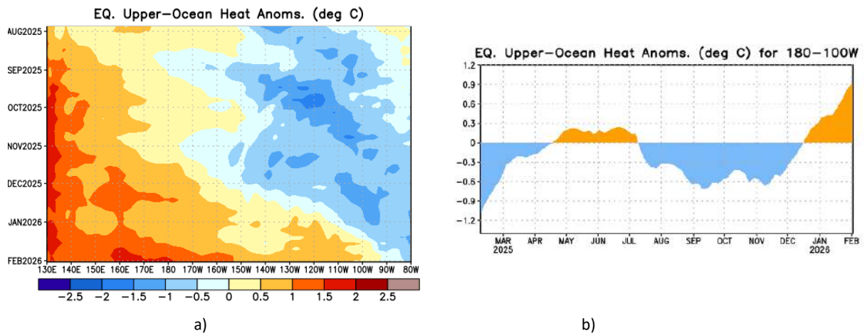
Figura 1.3.3 a) Anomalía del contenido de calor (°C) en el Pacífico ecuatorial (130°E-80°W), de 0m a 300 m de profundidad de agosto 2025 a enero 2026, y b) promedio del contenido de calor en la región ecuatorial entre 180°-100°W de febrero 2025 a enero 2026. Fuente: CPC-NOAA.
