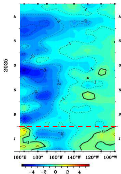
Figura 1.5.1. Diagrama Hovmöller de la anomalía del viento zonal a nivel del mar en el Pacífico ecuatorial. Periodo: agosto 2025 – enero 2026. Fuente: NOAA.
