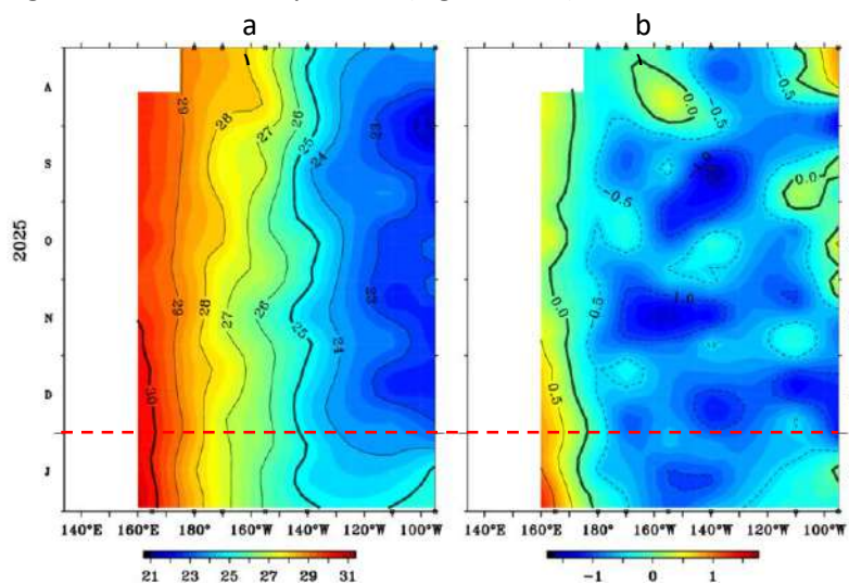
Figura 1.1.1 Diagrama Hovmöller de a) temperatura superficial del mar (TSM) (°C) y b) anomalía de TSM (°C) en el Pacífico ecuatorial (02°N - 02°S). Periodo: agosto 2025 – enero 2026. Fuente: TAO/TRITON, PMEL/NOAA.
