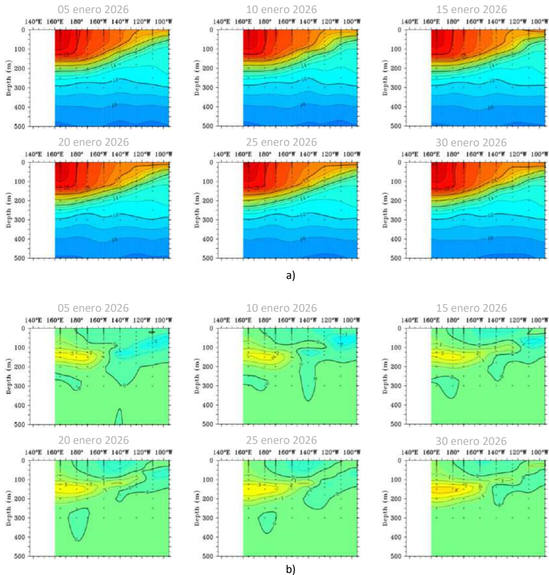
Figura 1.3.1. Sección transversal en el Pacífico ecuatorial (02°N - 02°S), promedio de cinco días, finalizando los días 5, 10, 15, 20, 25 y 30 de enero 2026 de la a) temperatura subsuperficial del mar (°C) y b) anomalía de la temperatura subsuperficial del mar (°C). Fuente: TAO/TRITON, PMEL/NOAA.
