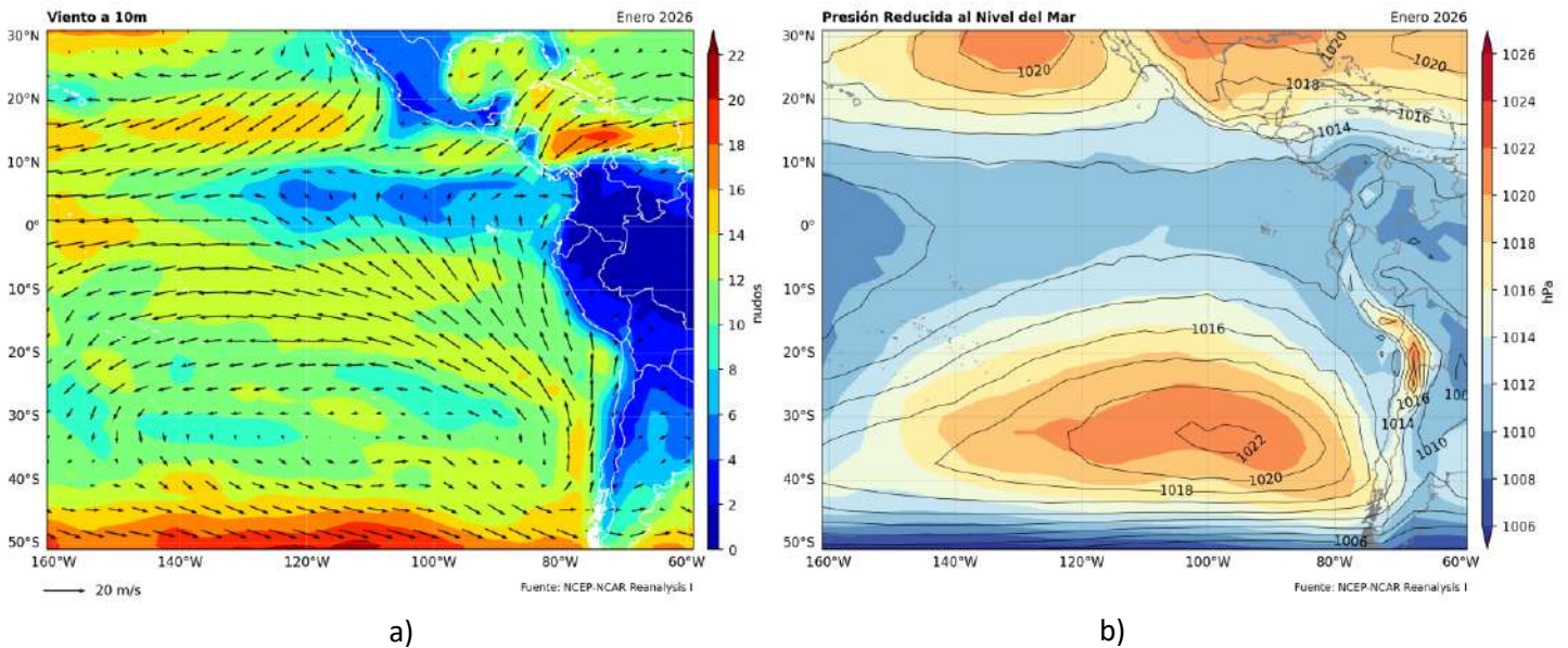
Figura 2.5.1. a) Circulación atmosférica a 10m de nivel del mar promedio (m/s) y b) presión al nivel del mar promedio (hPa), para enero 2026. Fuente: NCEP-NCAR Reanalysis. Procesamiento: DIHIDRONAV.
