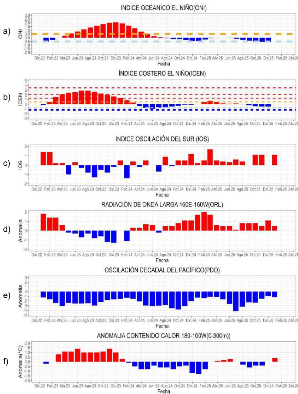
Figura 1.2.1 Índices climáticos a) ONI, b) ICEN, c) SOI (IOS), d) OLR, e) PDO y f) anomalía del contenido de calor 180-100W (0-300m). Climatología 1991- 2020. Fuente: NOAA, NCEI.
