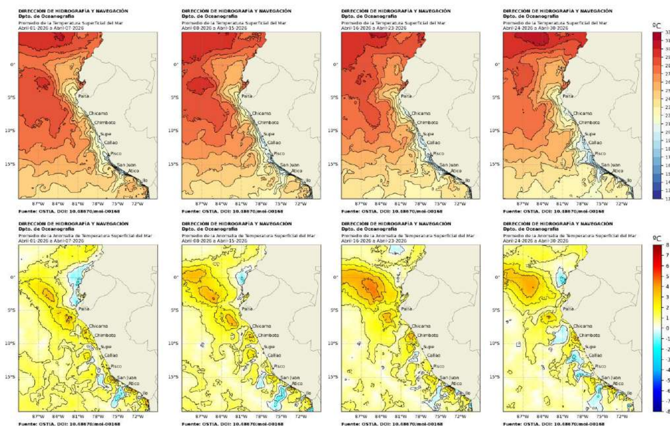
Figura 2.1.1. Promedios semanales de la temperatura superficial del mar y su anomalía ( ^{\circ}\text{C} ) en la región Niño 1+2 y frente a la costa de Perú para el mes de abril 2026. Fuente: OSTIA, Climatología: 1991–2020 (Pathfinder V5).
