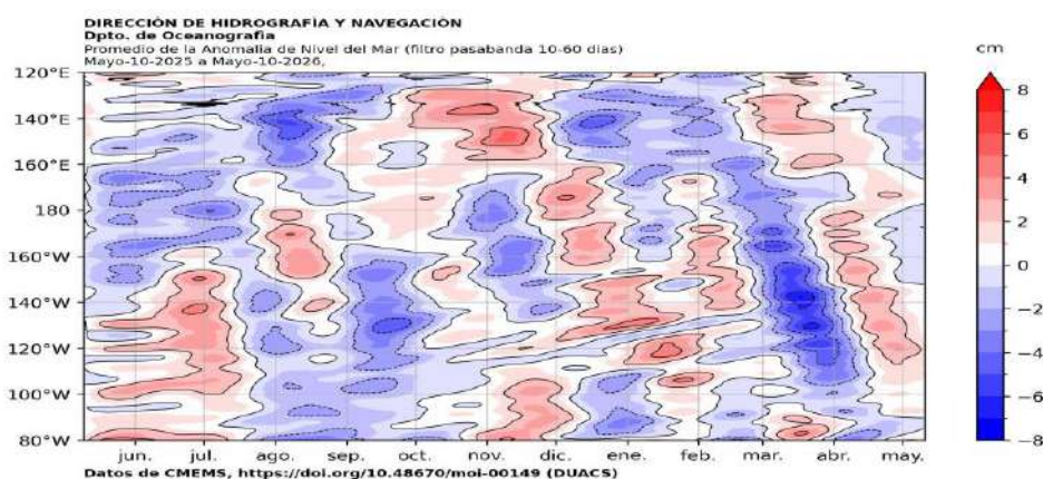
Figura 1.4.1. Diagrama de Hovmöller de la anomalía del nivel del mar en la región ecuatorial (cm), entre los 120°E-080°W (02°N - 02°S) con filtro pasa banda de 10-60 días. Periodo: 10 de mayo 2025 – 10 de mayo 2026. Fuente: GODAS, Climatología 1991–2020. Procesamiento: DIHIDRONAV.
