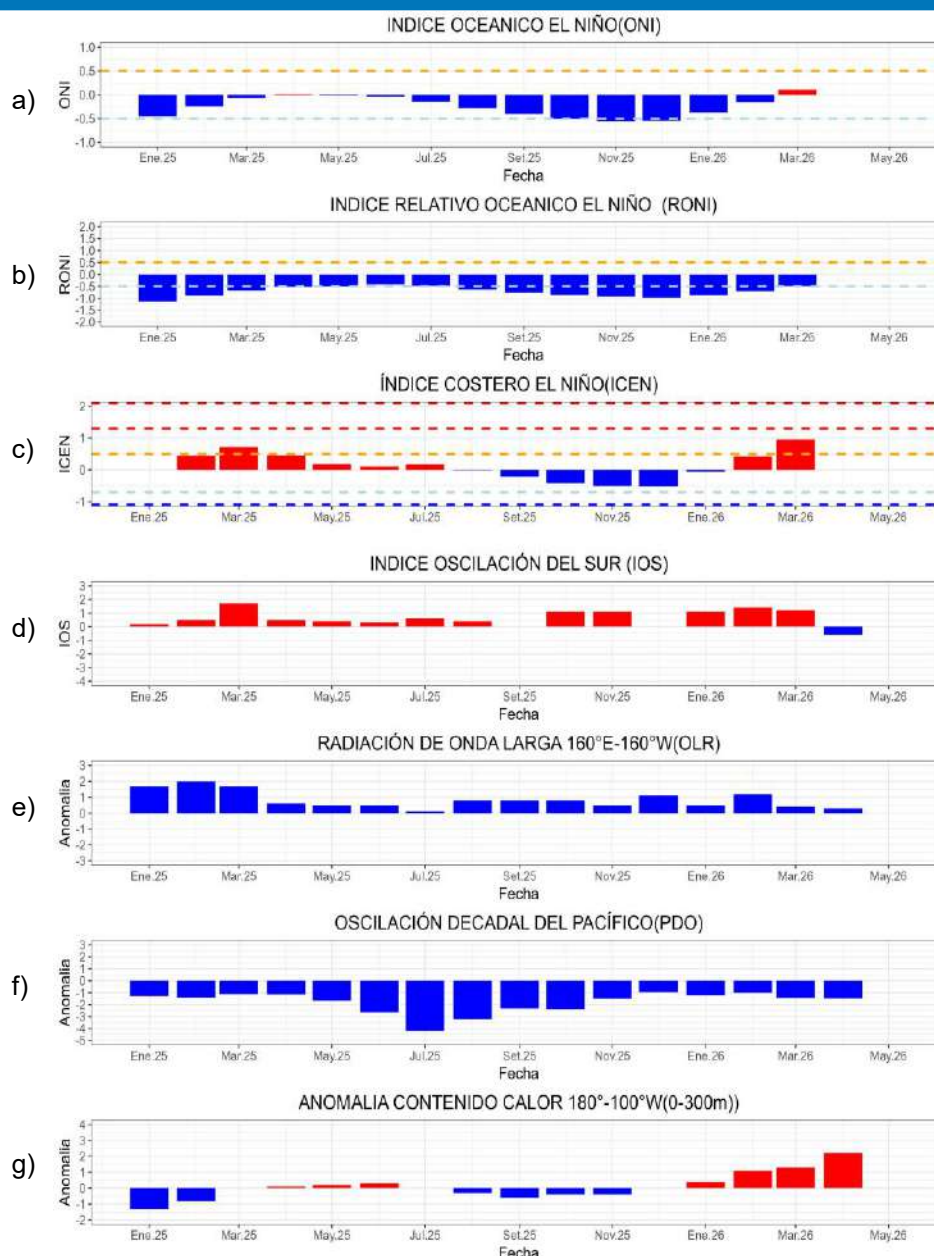
Figura 1.2.1 Índices climáticos a) ONI, b) RONI, c) ICEN, d) IOS, e) OLR, f) PDO y g) anomalía del contenido de calor 180-100W (0-300m). Climatología 1991- 2020. Fuente: NOAA, NCEI.
