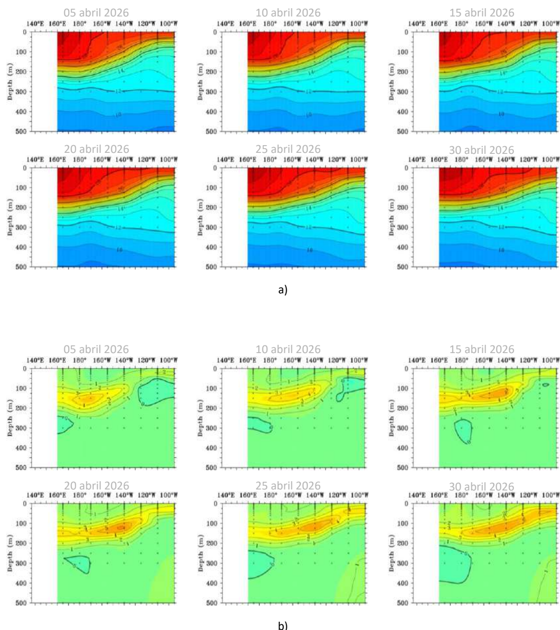
Figura 1.3.1. Sección transversal en el Pacífico ecuatorial (02°N - 02°S), promedio de cinco días, finalizando los días 5, 10, 15, 20, 25 y 30 de abril 2026 de la a) temperatura subsuperficial del mar (°C) y b) anomalía de la temperatura subsuperficial del mar (°C). Fuente: TAO/TRITON, PMEL/NOAA.
