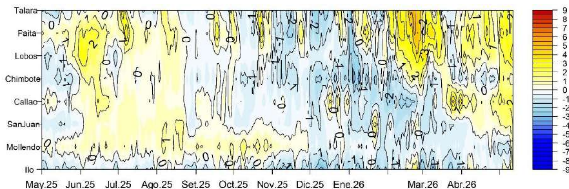
Figura 2.1.3. Diagrama Hovmöller de las anomalías de la TSM (°C) en el litoral de Perú. Periodo: mayo 2025 al 11 de mayo 2026. Climatología: 1991-2020. Fuente y procesamiento: DIHIDRONAV.
