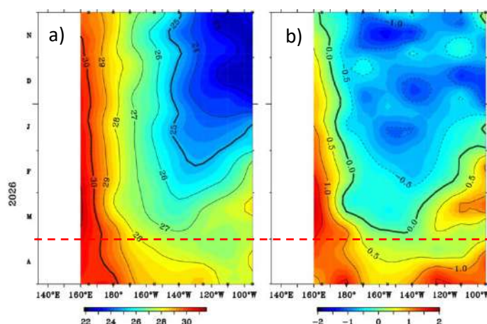
Figura 1.1.1 Diagrama Hovmöller de a) temperatura superficial del mar (TSM) (°C) y b) anomalía de TSM (°C) en el Pacífico ecuatorial (02°N - 02°S). Periodo: noviembre 2025 – abril 2026. Fuente: TAO/TRITON, PMEL/NOAA.
