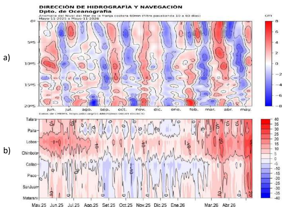
Figura 2.4.1. Diagrama Hovmöller de la anomalía del nivel del mar (cm) a) promedio entre 60 millas en la costa de Ecuador y Perú (02°N - 20°S), con periodo mayo 2025 - 11 de mayo 2026, y b) en el litoral de Perú, con periodo mayo 2025 al 11 de mayo 2026. Fuente: CMEMS/Mercator y DIHIDRONAV. Procesamiento: DIHIDRONAV.
