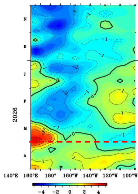
Figura 1.5.1. Diagrama Hovmöller de la anomalía del viento zonal a nivel del mar en el Pacífico ecuatorial. Periodo: noviembre 2025 – abril 2026. Fuente: NOAA.
