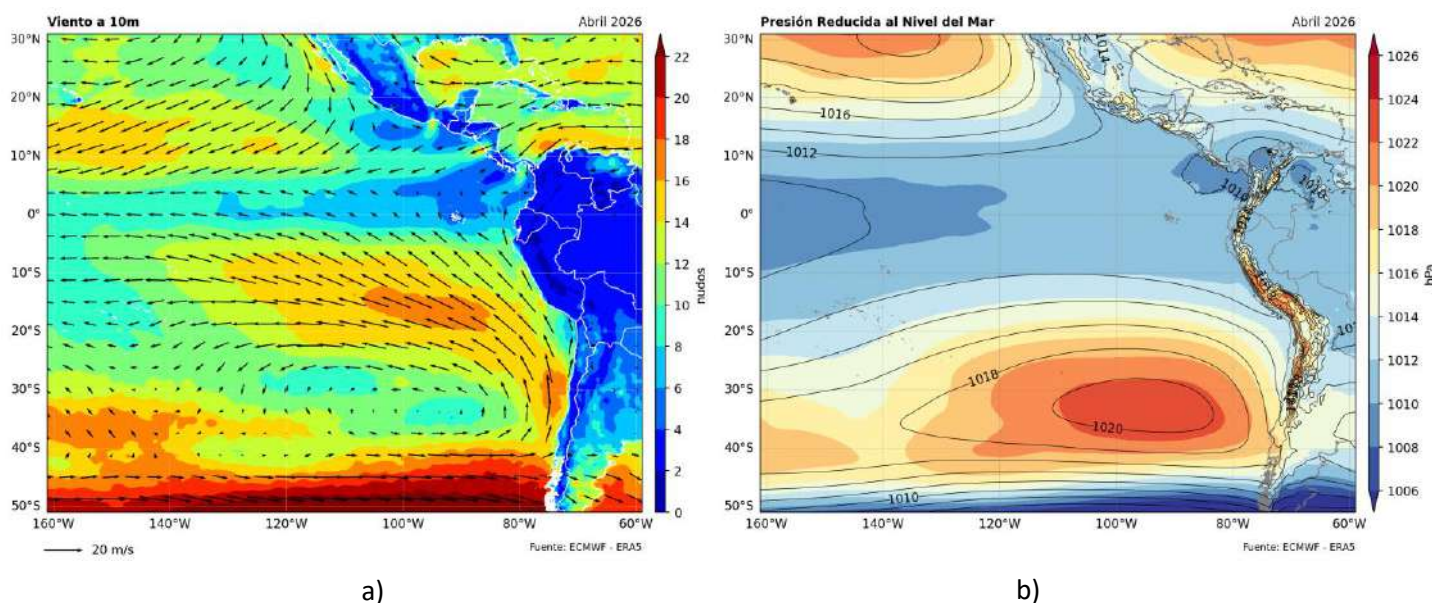
Figura 2.5.1. a) Circulación atmosférica a 10m de nivel del mar promedio (m/s) y b) presión al nivel del mar promedio (hPa), para abril 2026. Fuente: NCEP-NCAR Reanalysis. Procesamiento: DIHIDRONAV.
