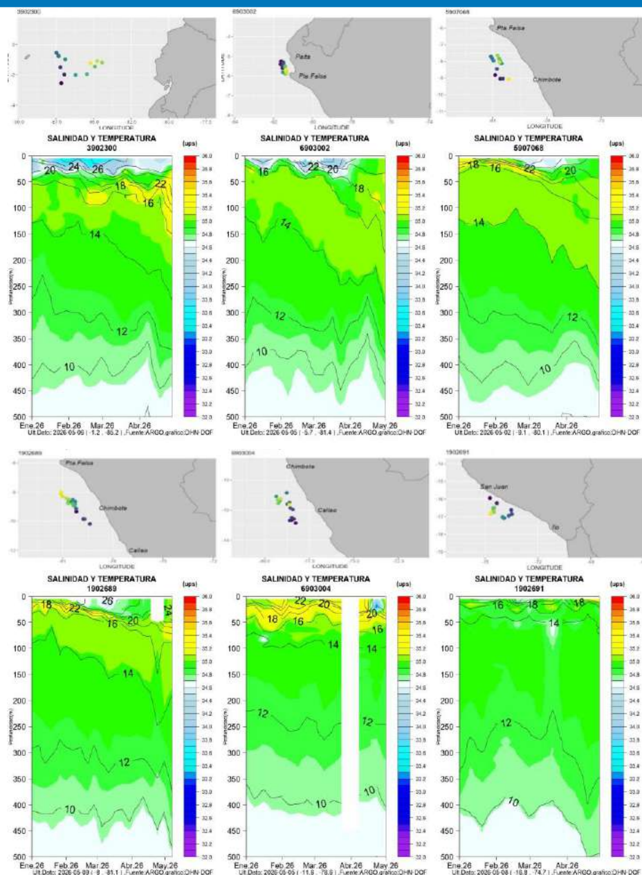
Figura 2.3.2. Secciones de salinidad del mar con profundidad de las isotermas (Contornos) de enero 2026 a mayo 2026 hasta los 500 m de profundidad. Fuente: ARGO. Procesamiento: DIHIDRONAV.
