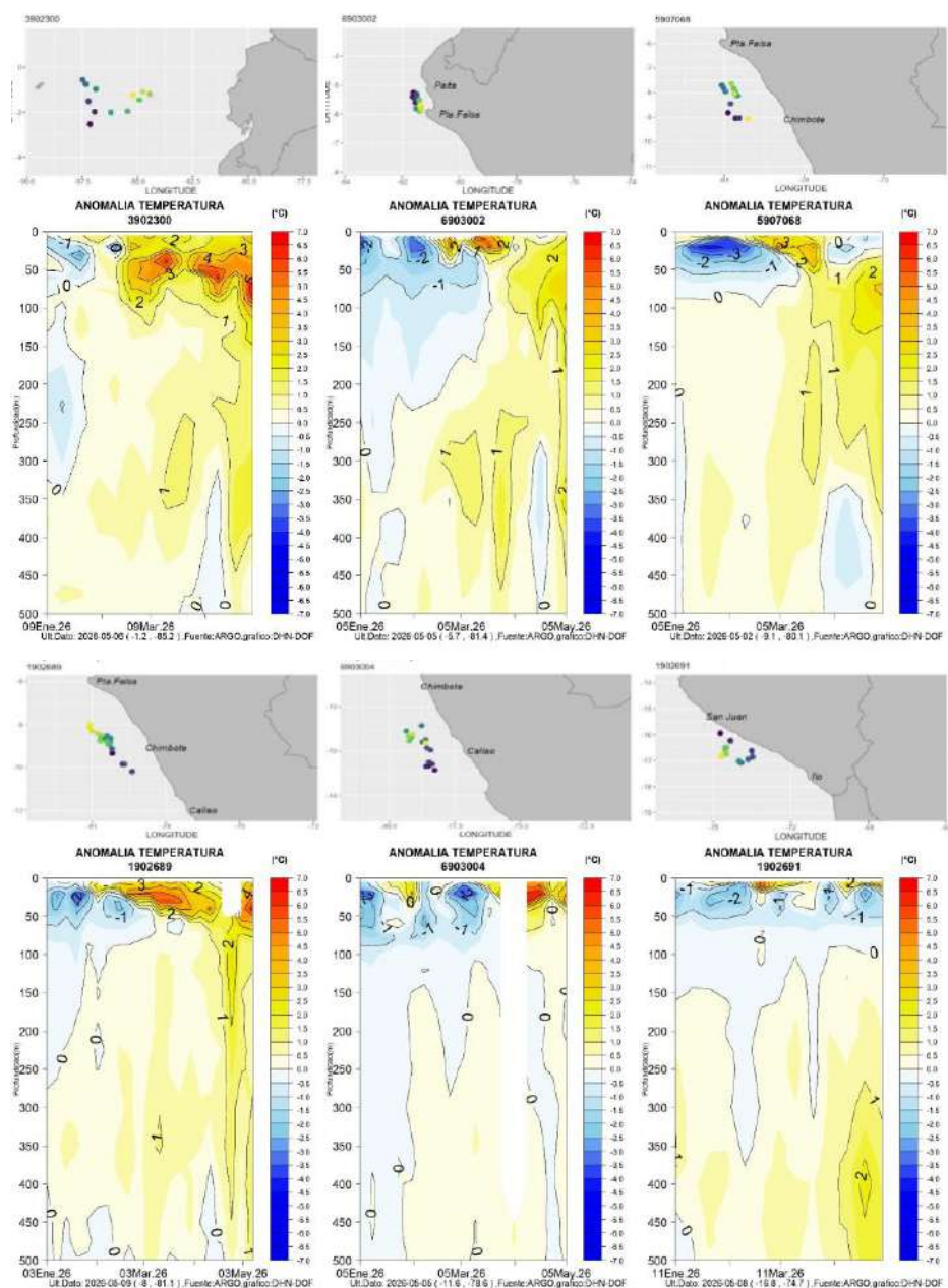
Figura 2.2.1. Secciones de anomalía de temperatura del mar de enero 2026 a mayo 2026 hasta los 500 m de profundidad. Fuente: ARGO. Procesamiento: DIHIDRONAV.
