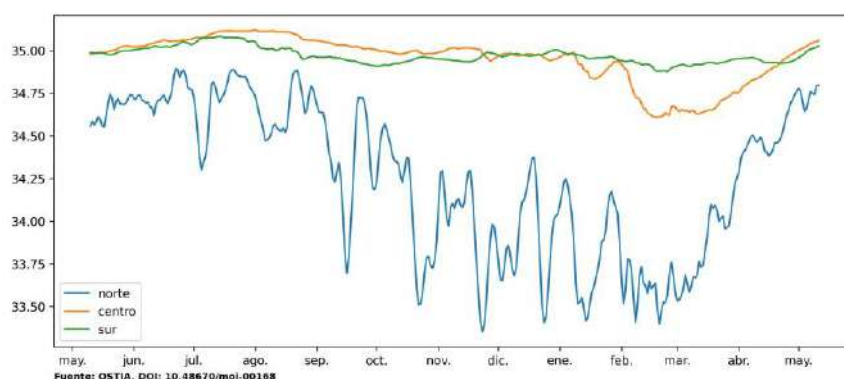
Figura 2.3.1. Promedio diario de la salinidad superficial del mar dentro de las primeras 60mn frente a la costa de Perú del 10 de mayo de 2025 al 11 de mayo de 2026. Fuente MERCATOR. Procesamiento: DIHIDRONAV.
