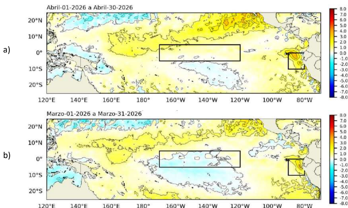
Figura 1.1.3 Promedio mensual de la anomalía de la temperatura superficial del mar (°C) del mes de a) abril 2026 y b) marzo 2026. Fuente: OSTIA, Climatología 1991–2020. Procesamiento: DIHIDRONAV.
